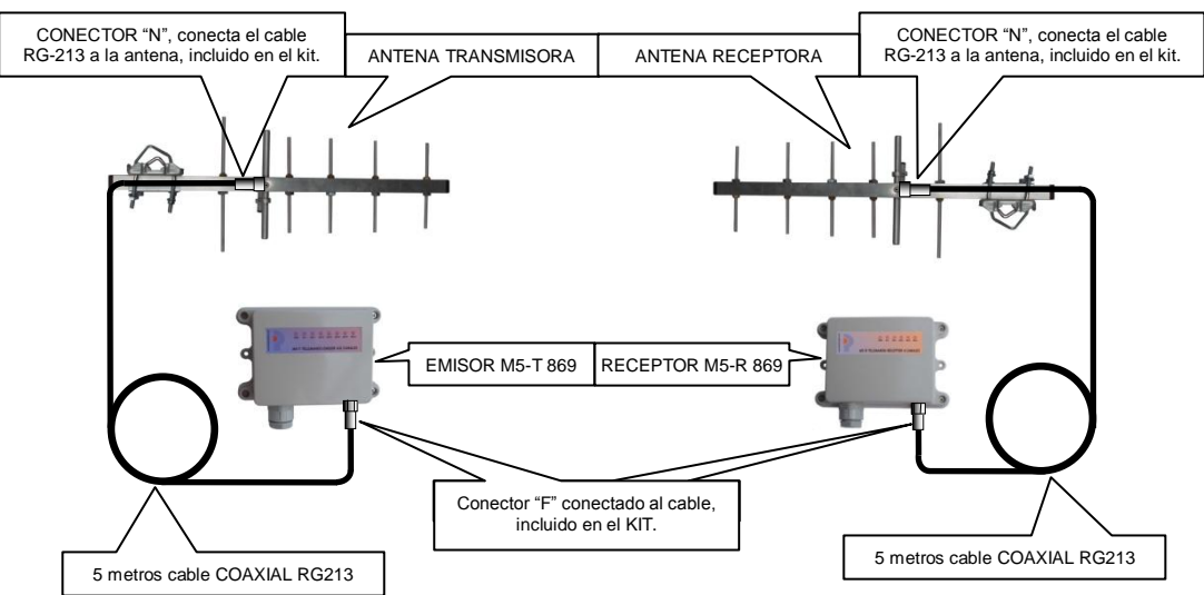
Fig 3. Cableado i conexión de los equipos a las antenas.
