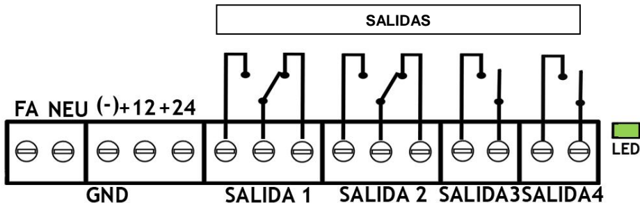
FIG-2. CONEXIONADO SALIDAS.
