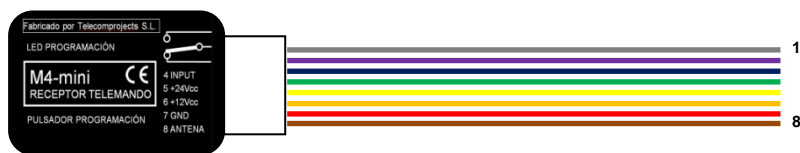
Fig 1, el telemando receptor M4-Mini dispone de un conector con 8 conexiones.
