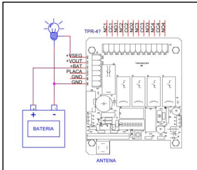
Fig 2 conexionado salida relé de cortésia o de seguridad. Al activar cualquiera de los relés 1,2,3 o 4, el relé de seguridad permanecerá activado y la luz se encenderá.
